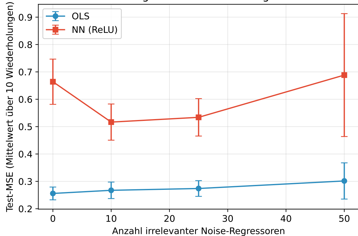
MSE-Anstieg durch irrelevante Regressoren
