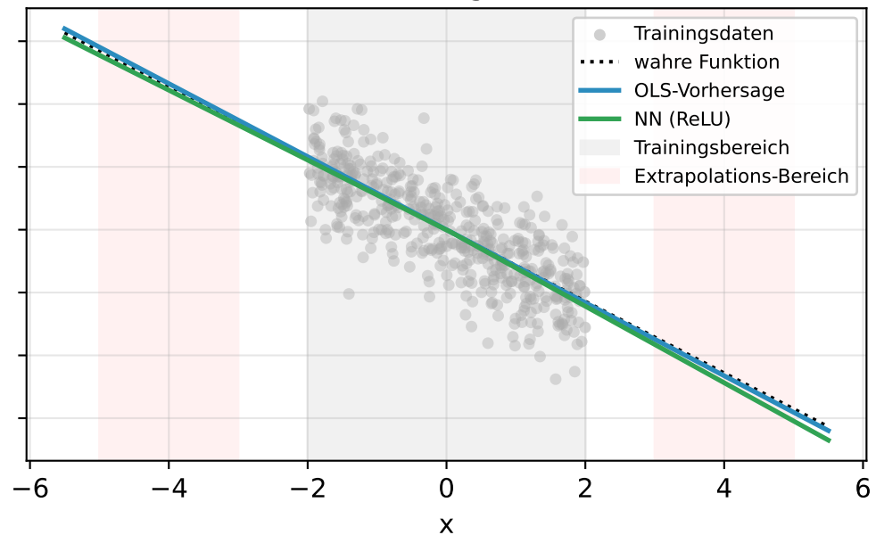
Aktivierung: ReLU
