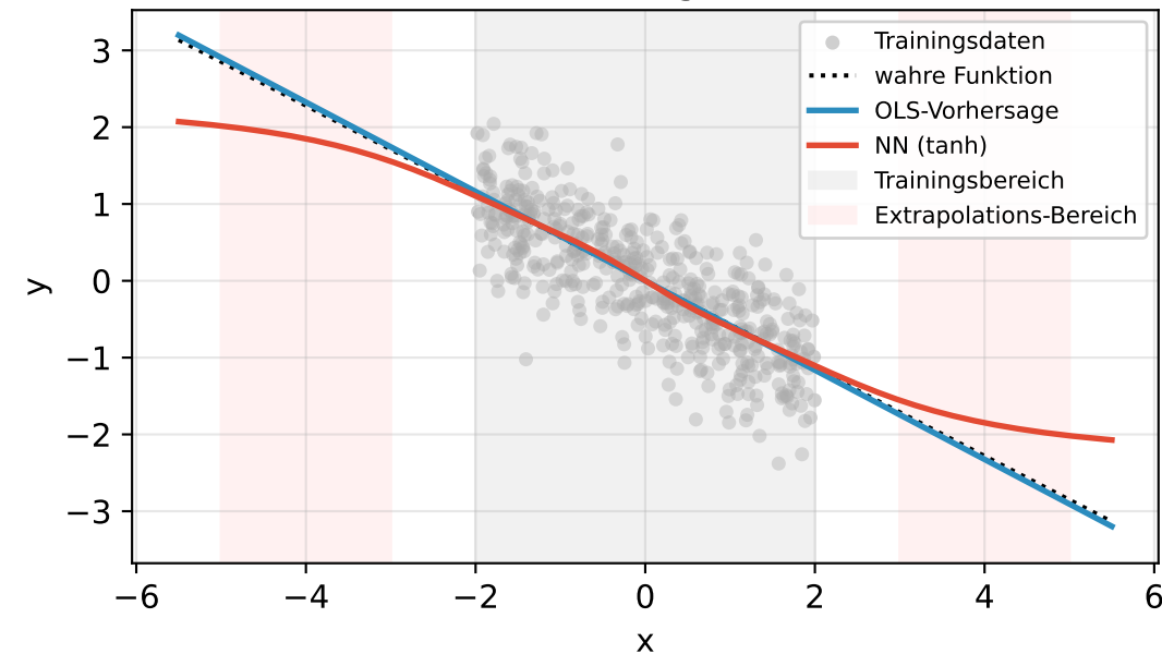
Aktivierung: tanh
