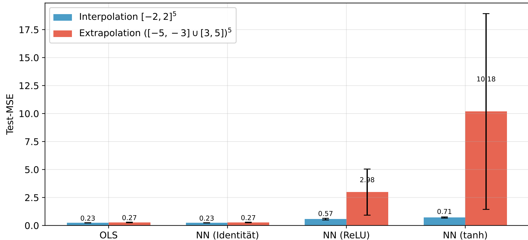
Test-MSE in Interpolations- und Extrapolationsbereich ( p = 5, 10 Seeds)
