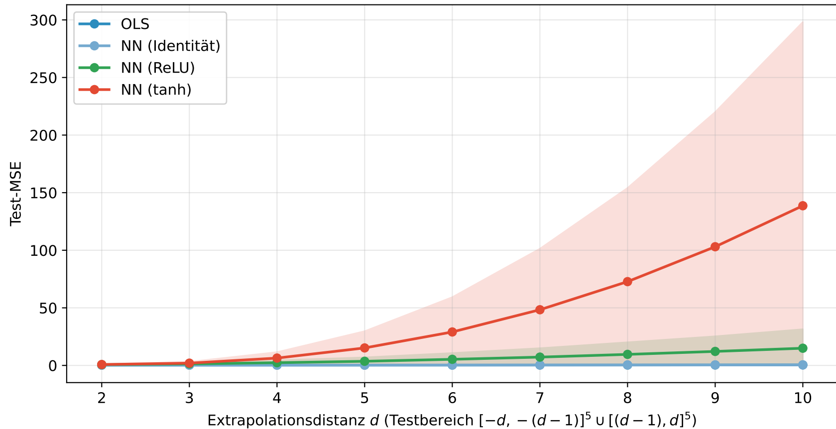
Test-MSE über Extrapolationsdistanz ( p = 5, 10 Seeds)
