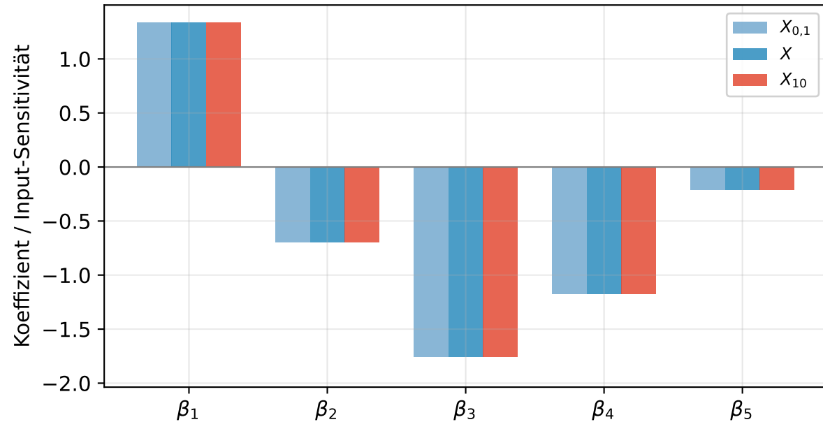
OLS: zurückskalierte Koeffizienten
