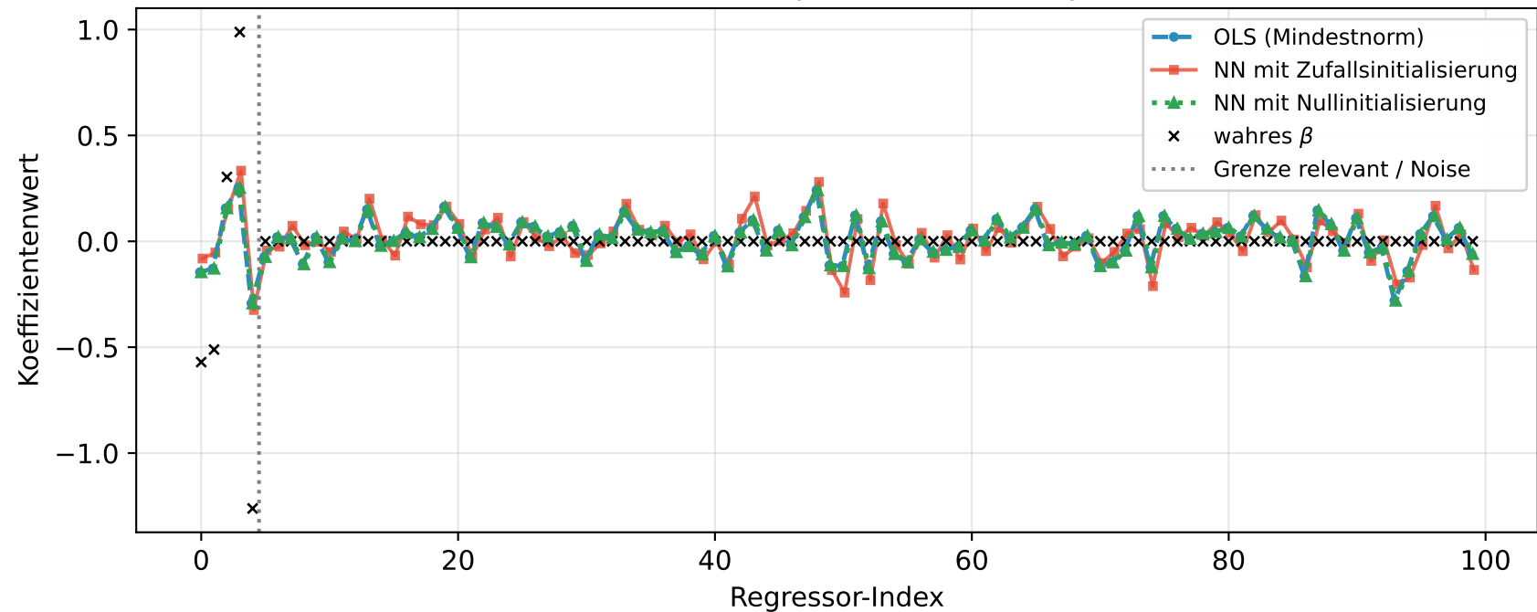
Koeffizientenprofile im Fall n < p
