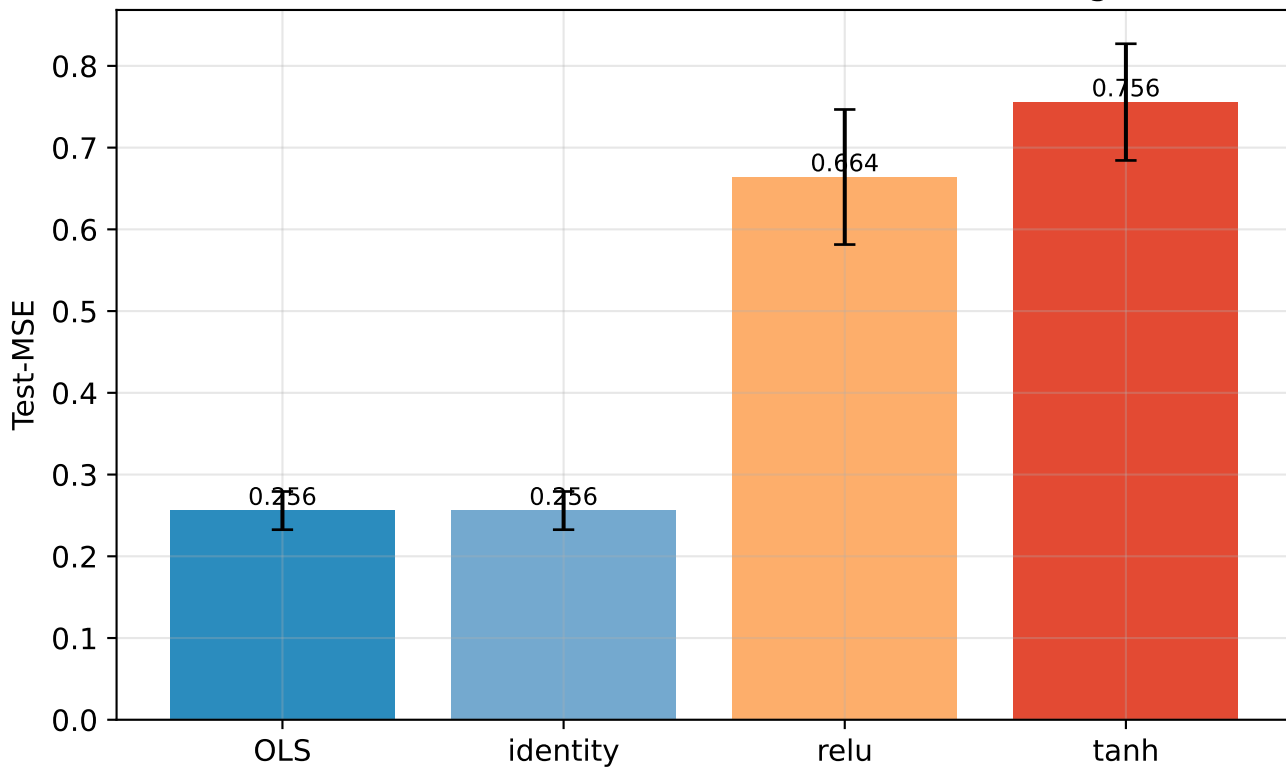
Test-MSE über 10 Seeds: OLS vs. NN-Aktivierungen
