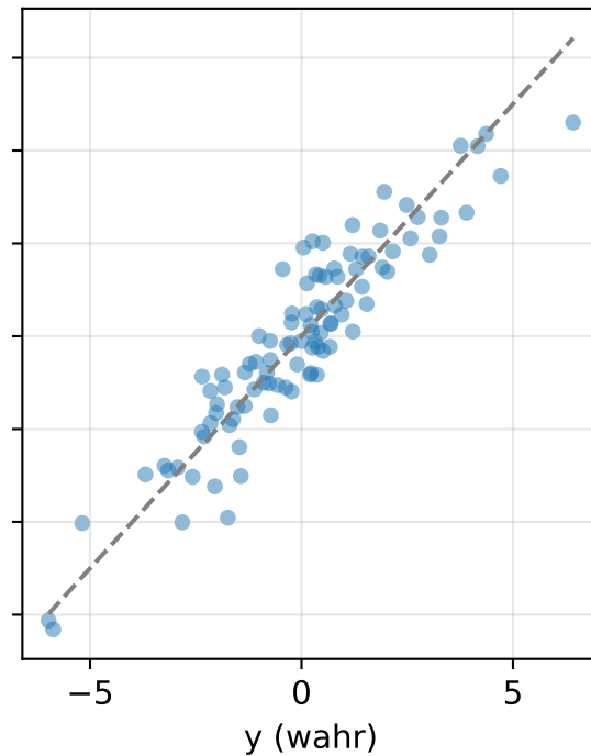
relu (MSE=0.651)
