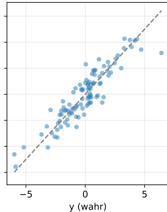
tanh (MSE=0.771)
