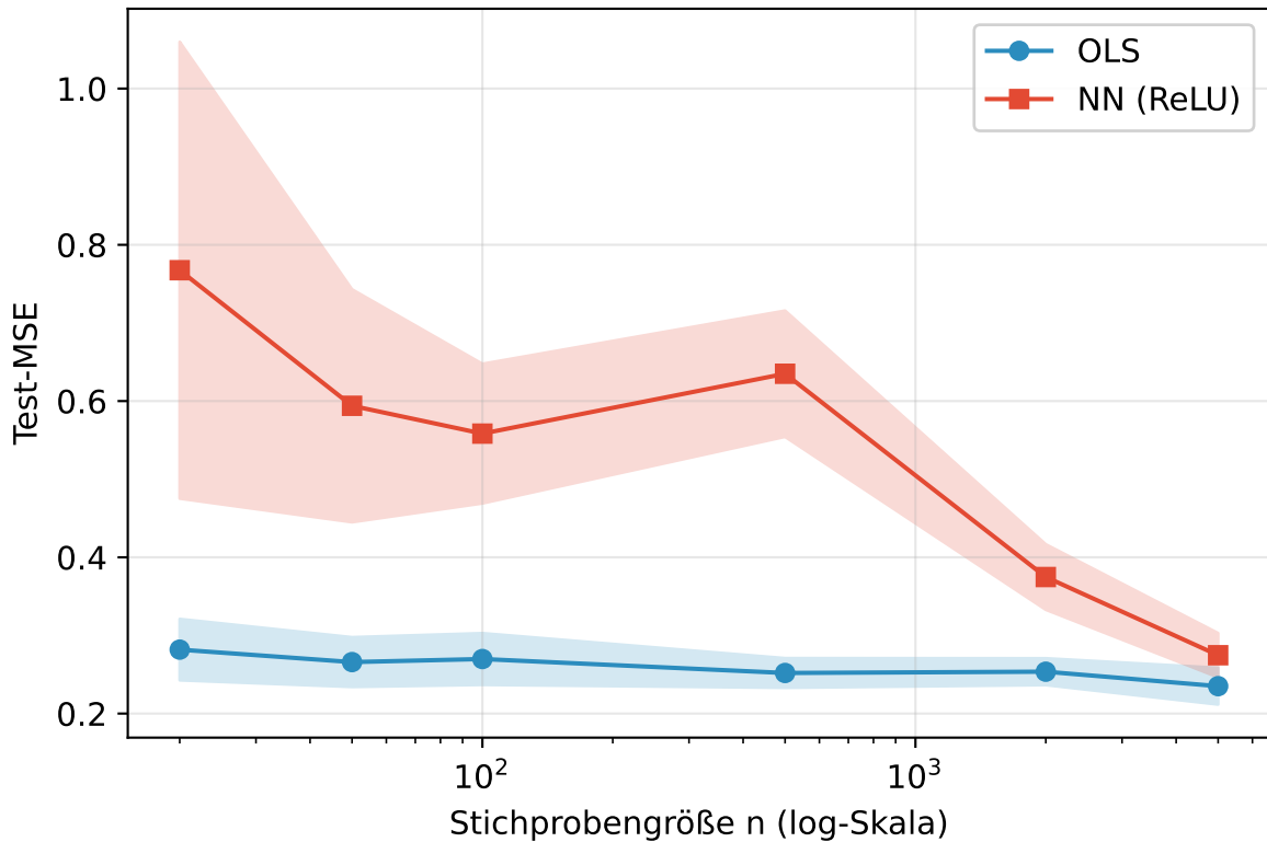
Lernkurve: Test-MSE über n
