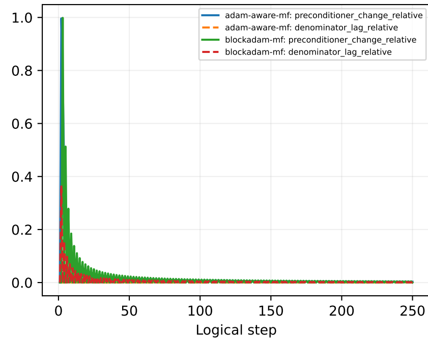
cv: DP preconditioner changes and lag
