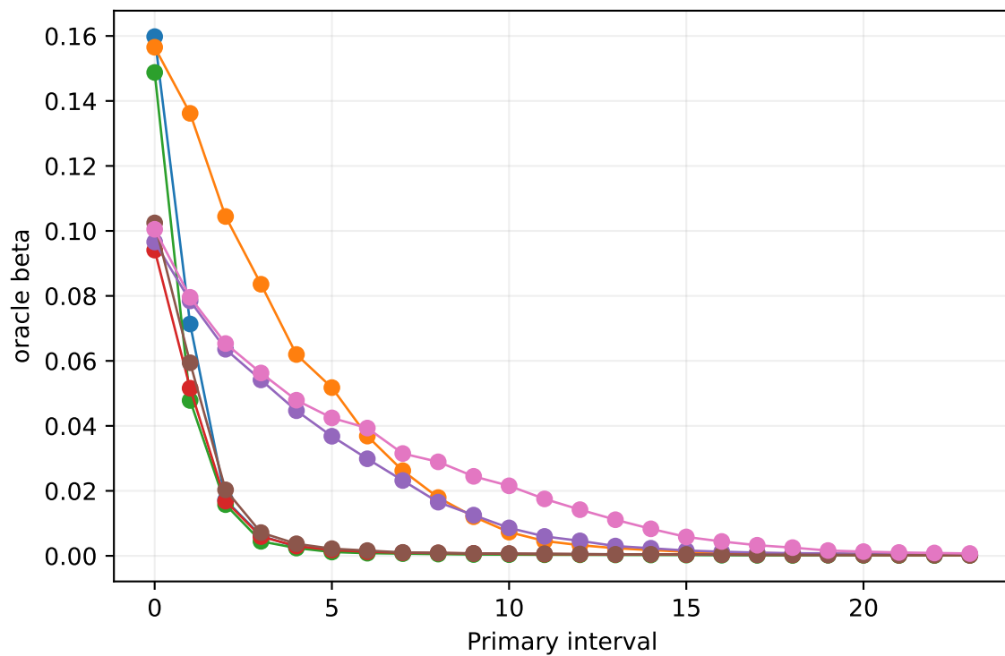
fc1
