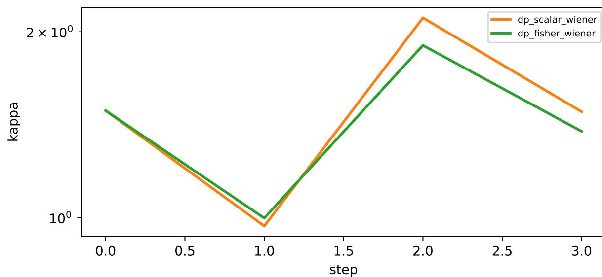
conv2
