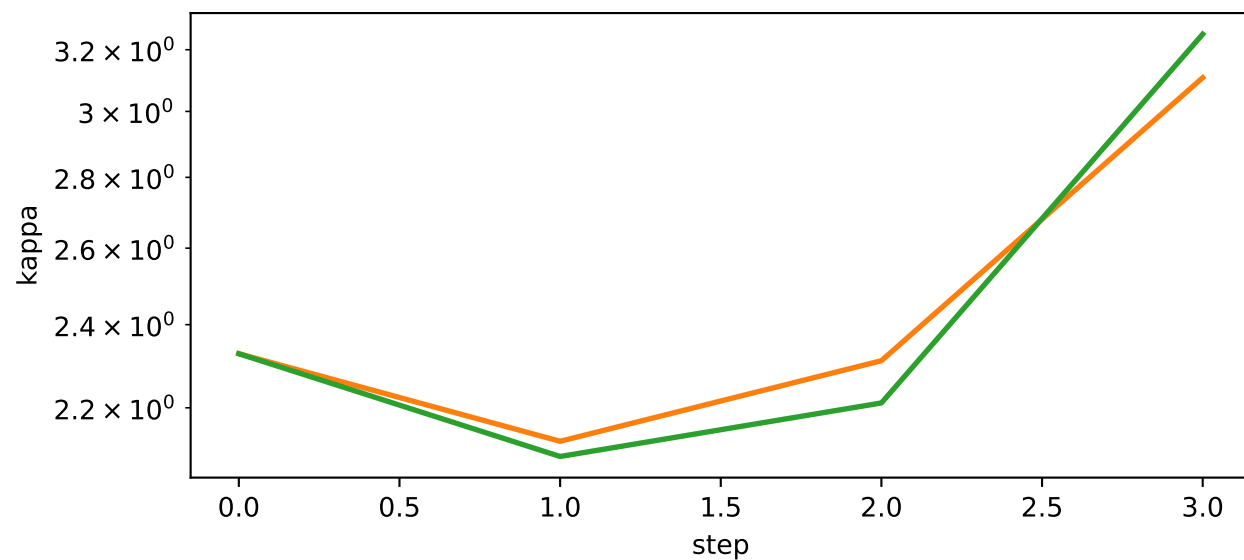
fc1
