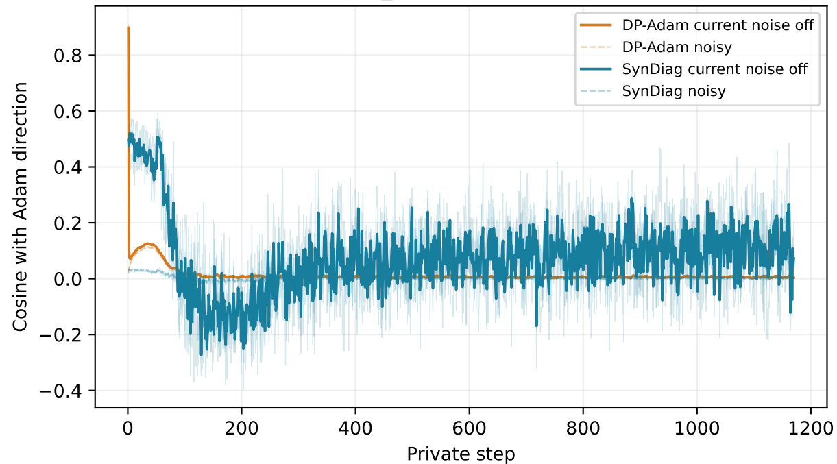
dp_adam trajectory
