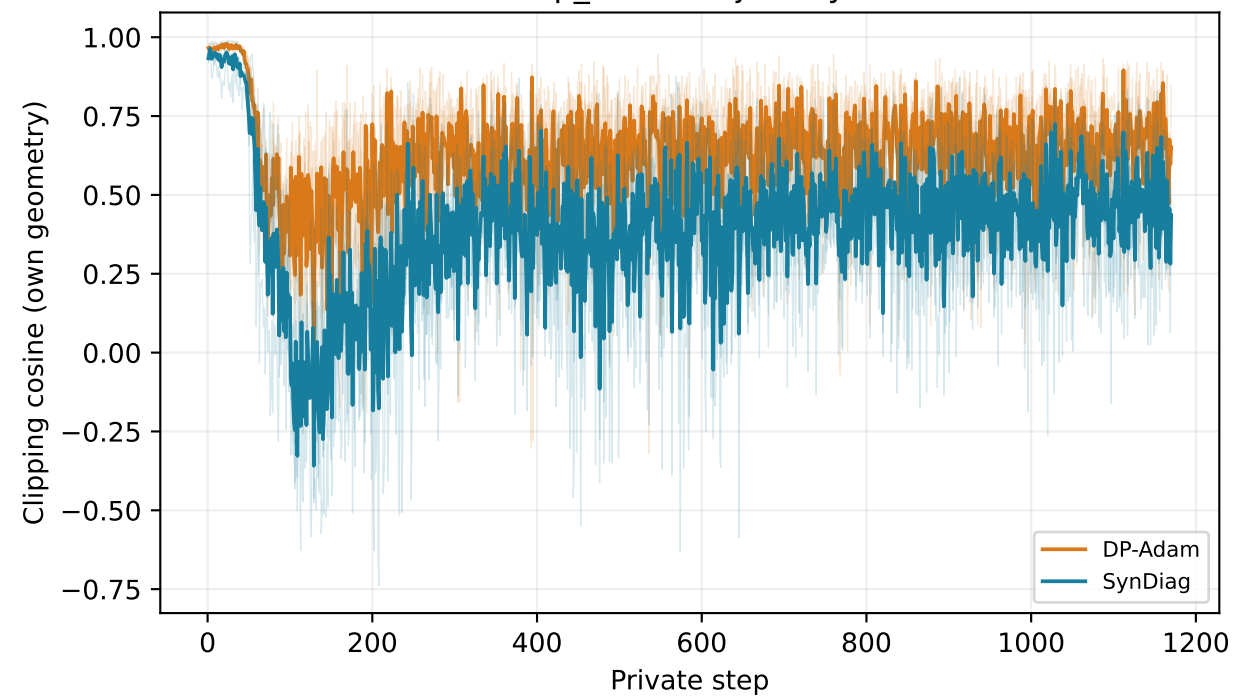
dp_adam trajectory
