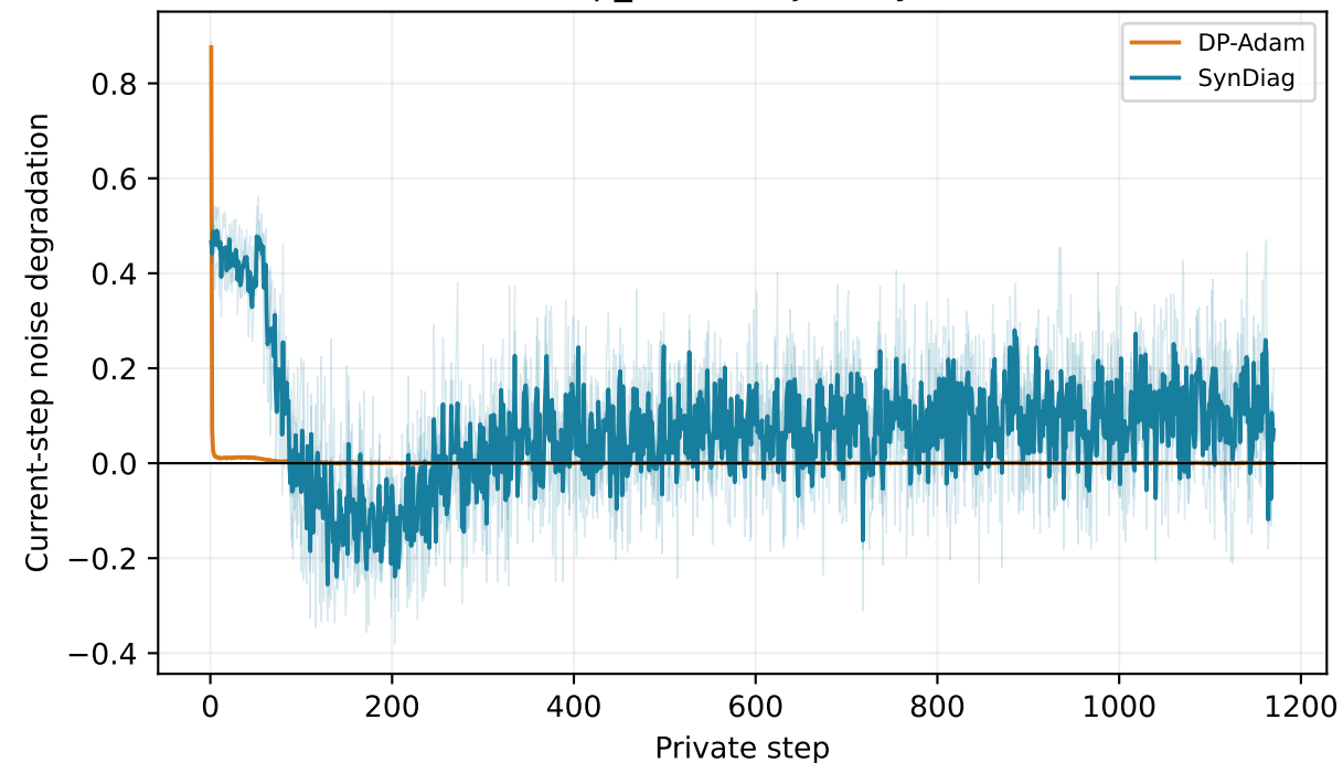
dp_adam trajectory
