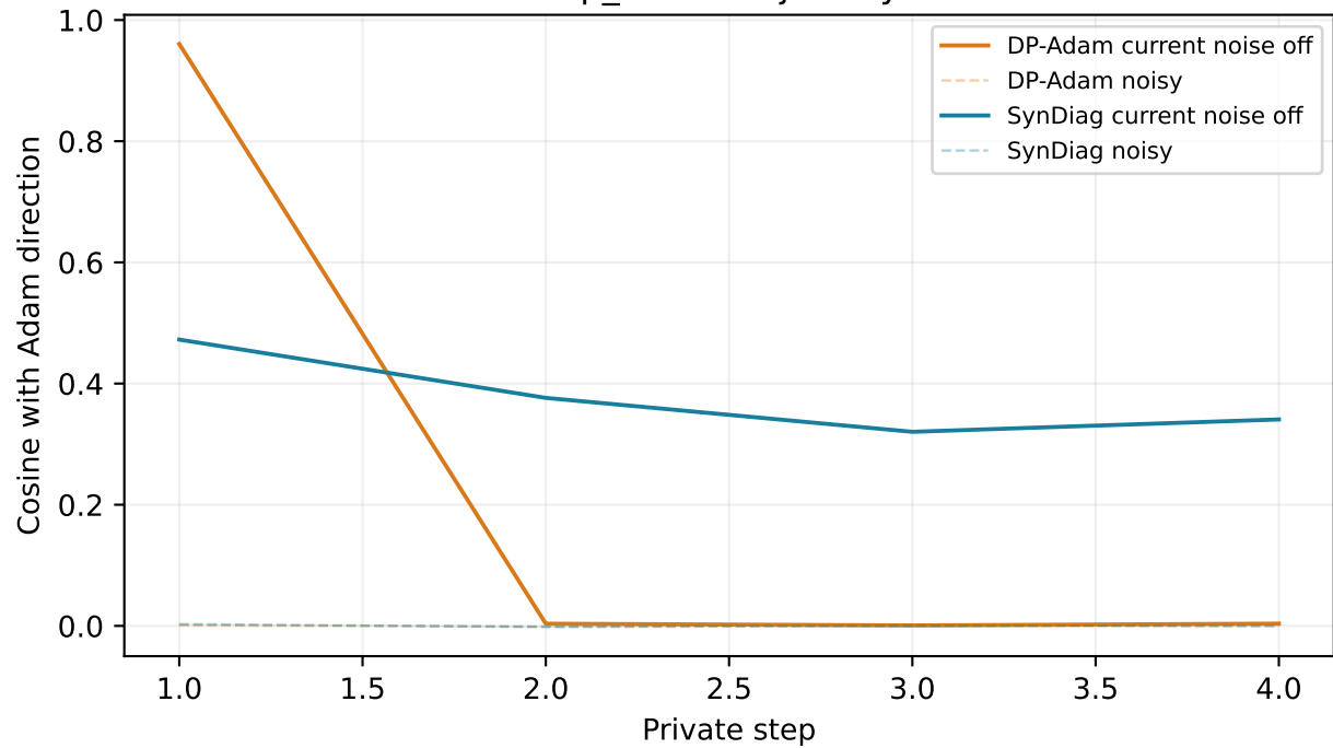
dp_adam trajectory
