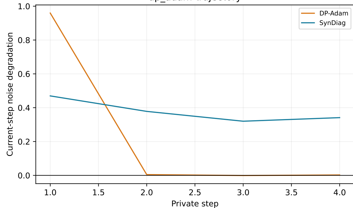
dp_adam trajectory
