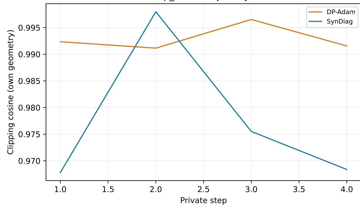
dp_adam trajectory
