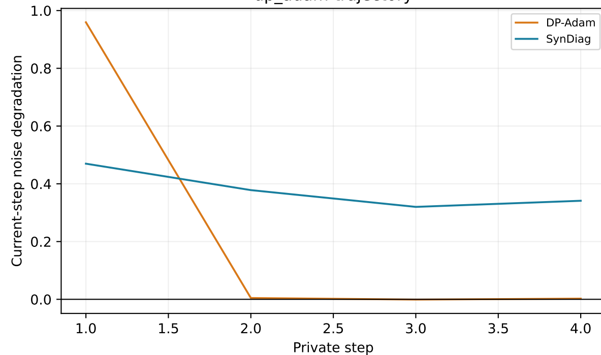
dp_adam trajectory
