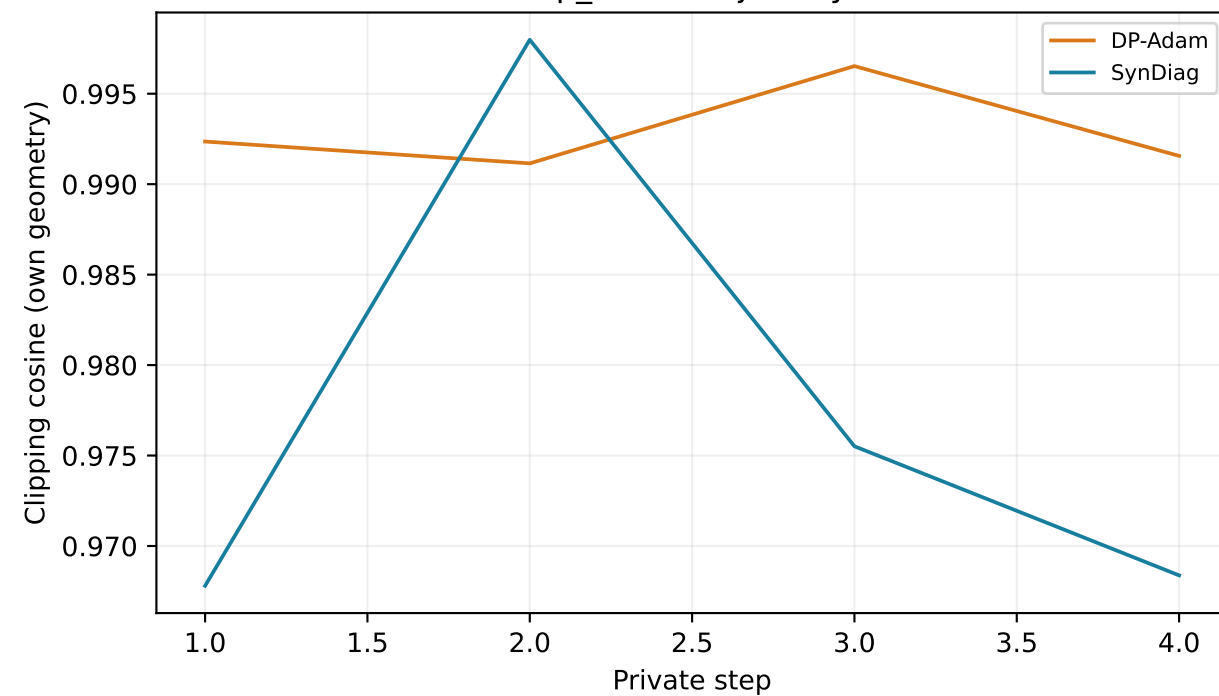
dp_adam trajectory
