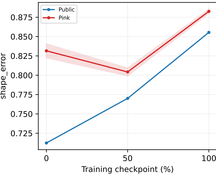
conv1
