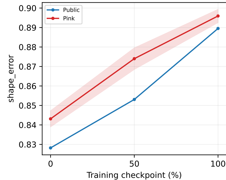
fc1
