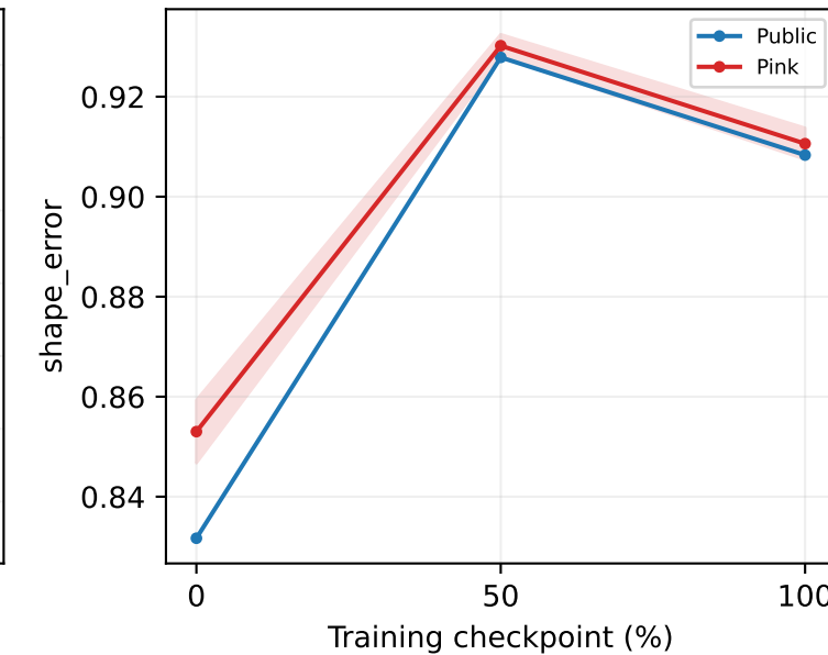
conv2
