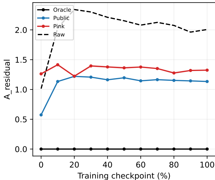
conv1
