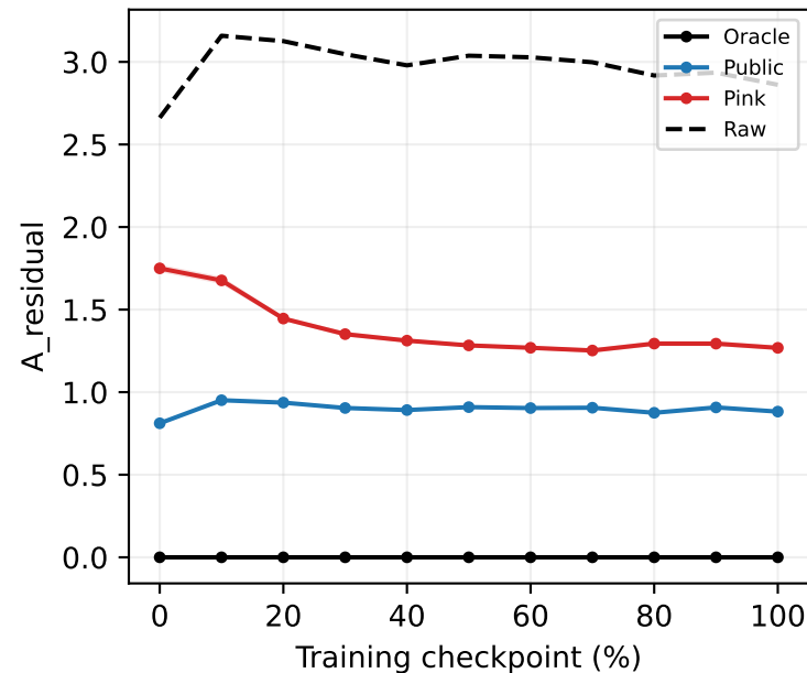
conv2
