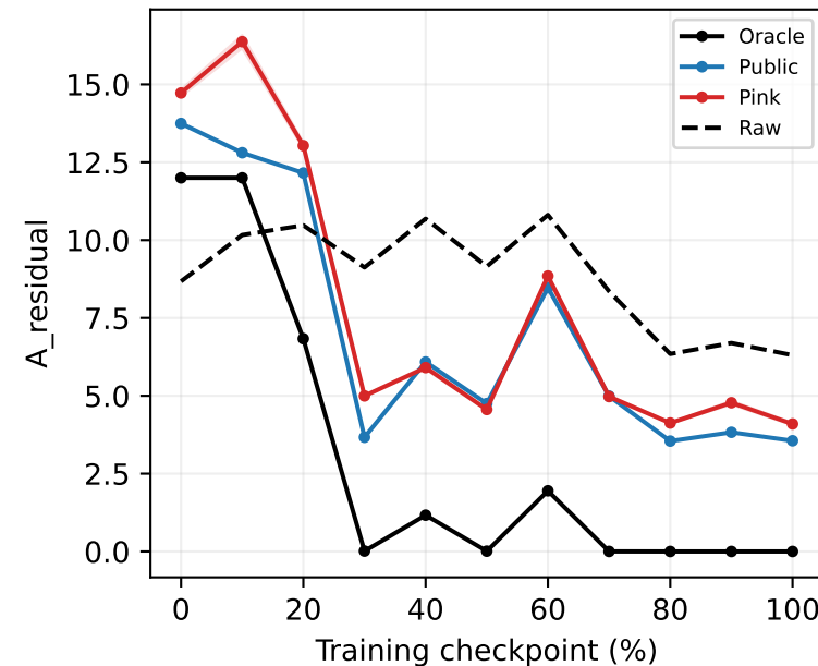
fc1
