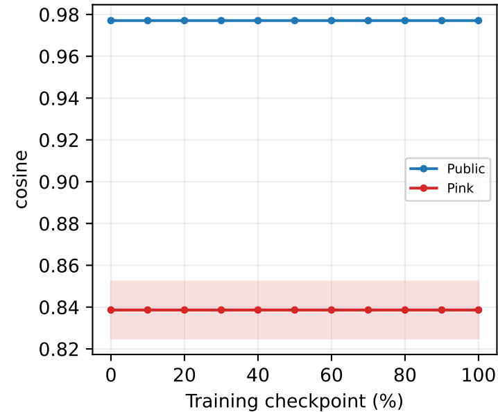
conv1: cos(G) [raw]
