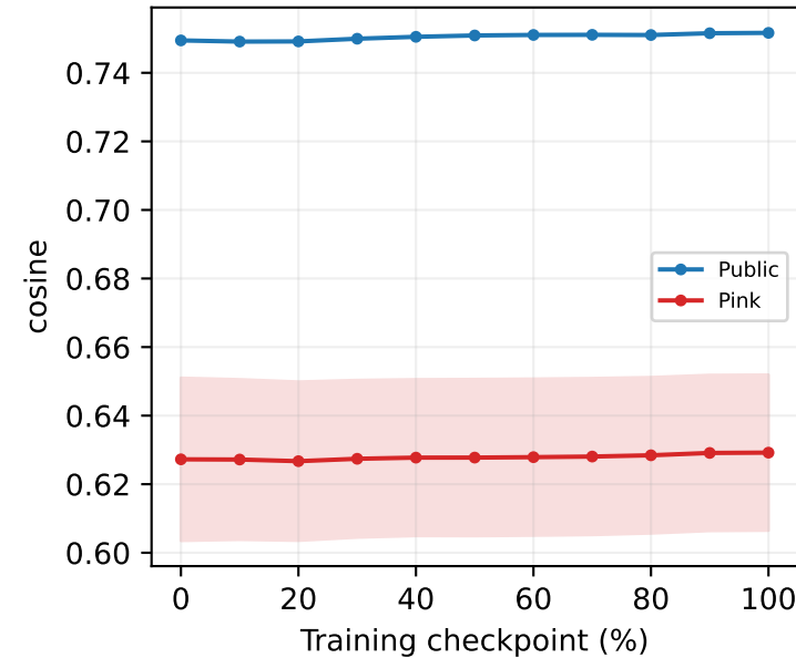
fc1: cos(G) [raw]
