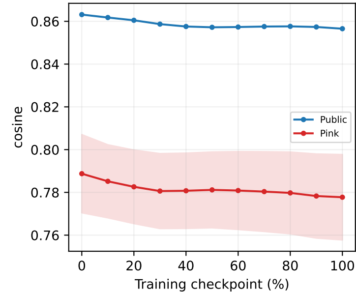
fc2: cos(G) [raw]
