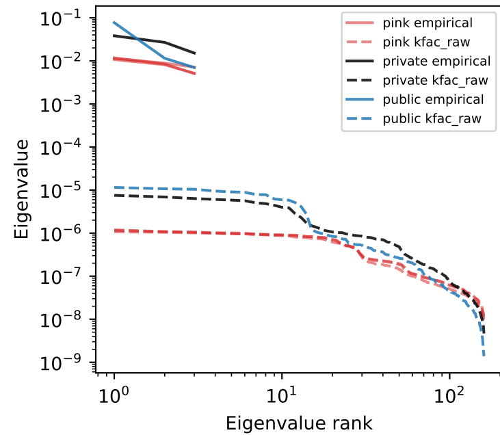
conv1 / 50%
