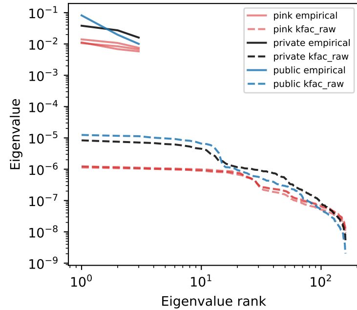
conv1 / 100%
