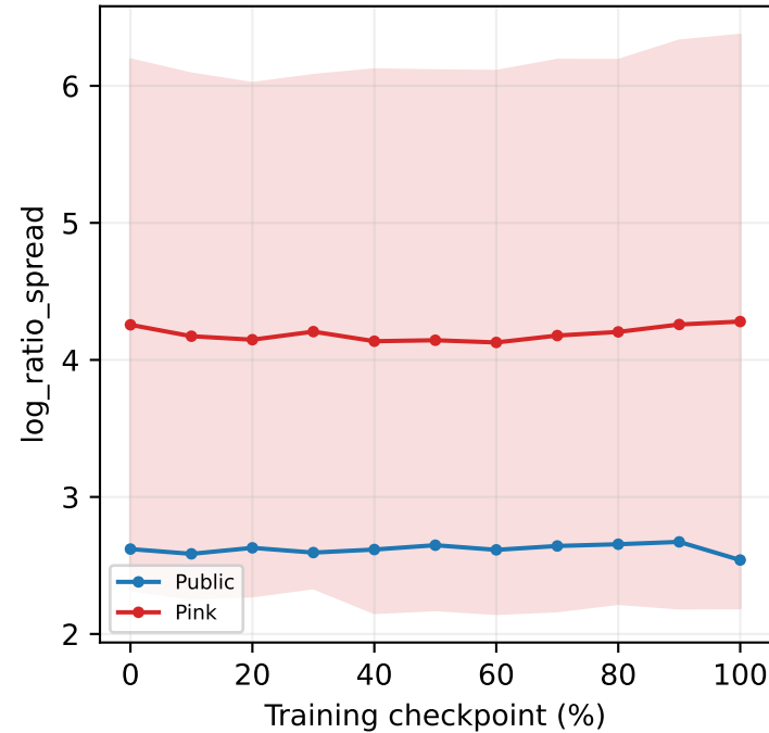
conv2
