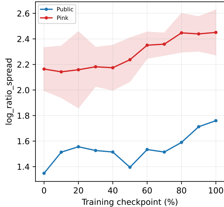
conv1
