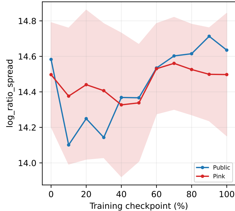
fc1
