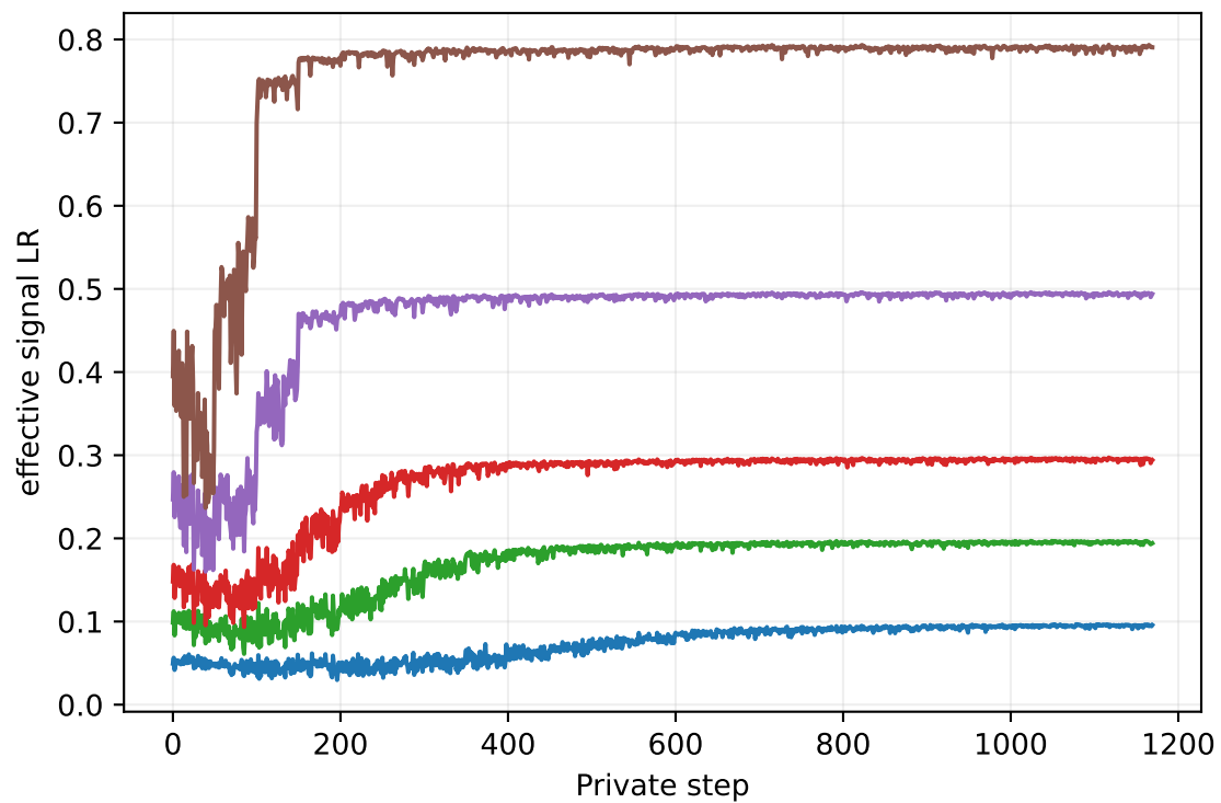
fc1
