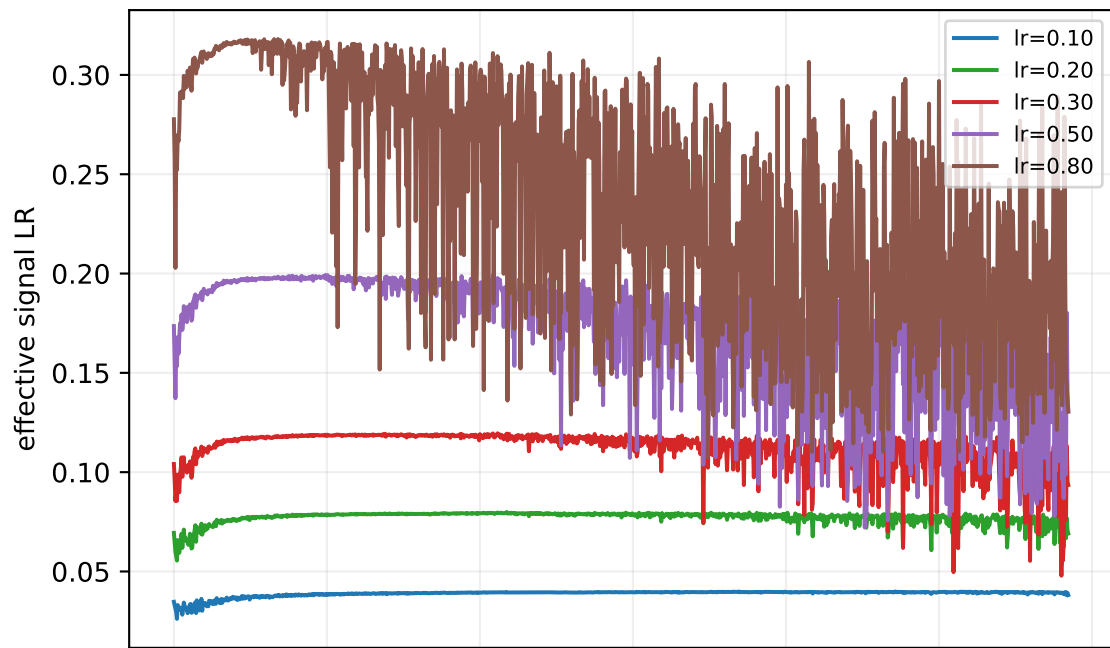
conv1
