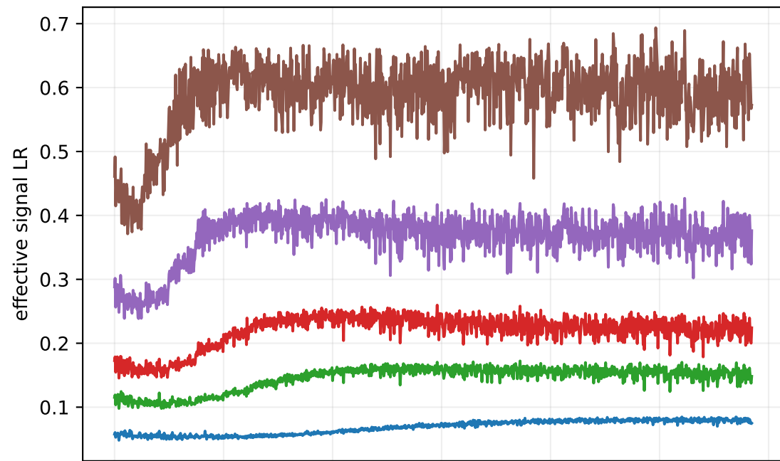
conv2
