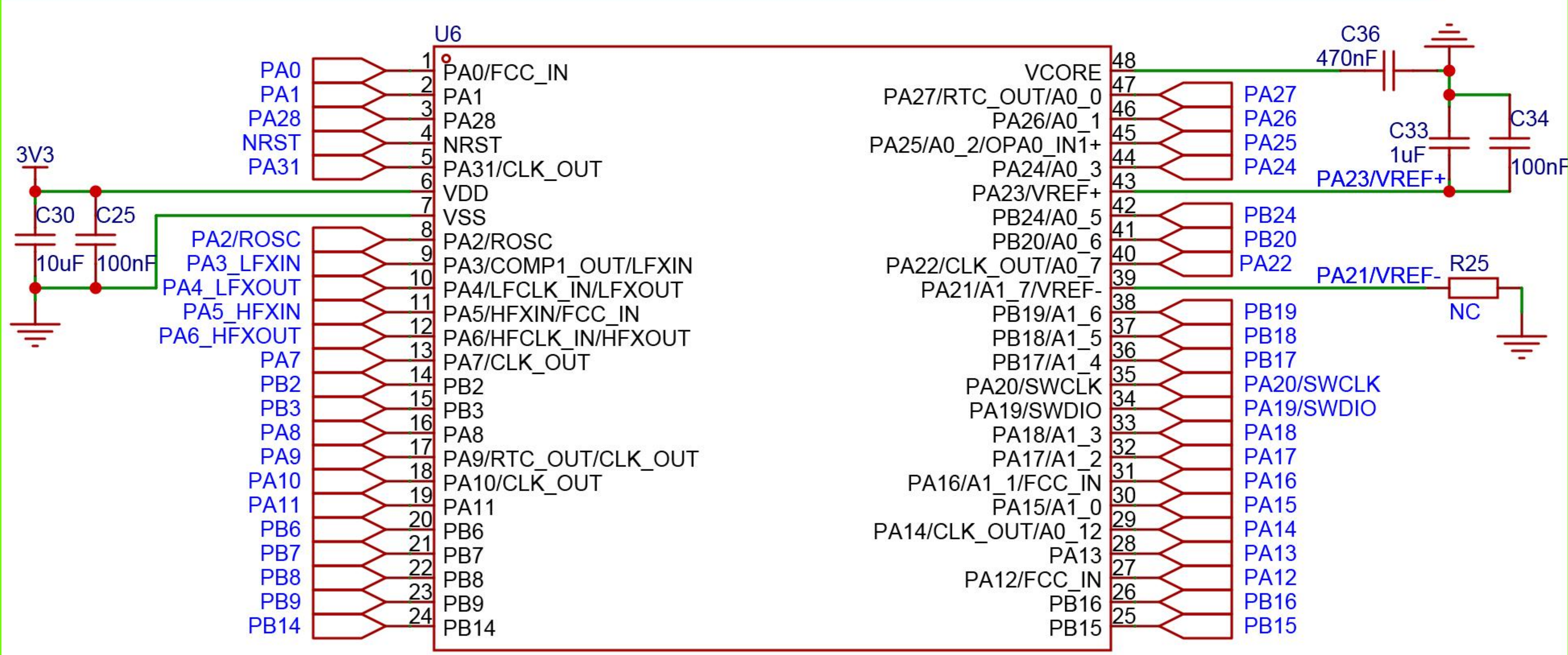
主控MSPM0G3507
