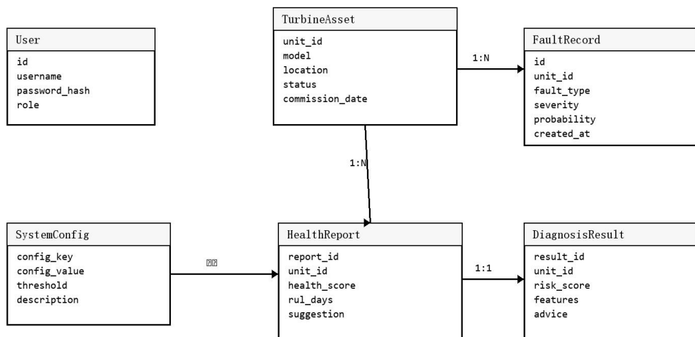
齿轮箱健康管理系统ER图
