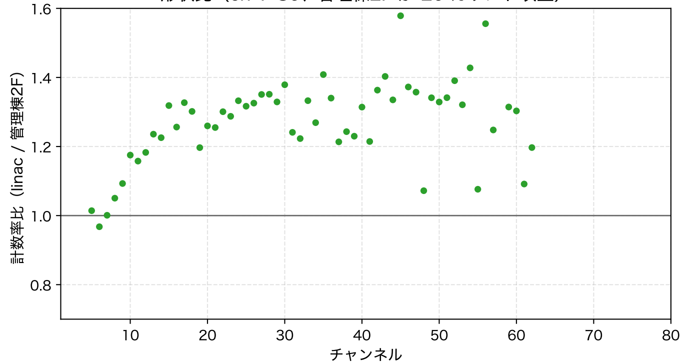
形状比 (ch 1-80、管理棟2F が 20 カウント以上)
