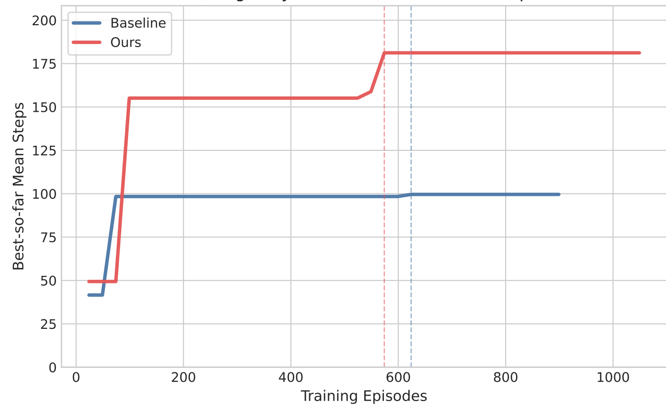
(d) Highway Dense: Best-so-far Envelope
