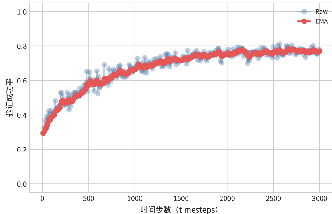
单种子验证收敛曲线
