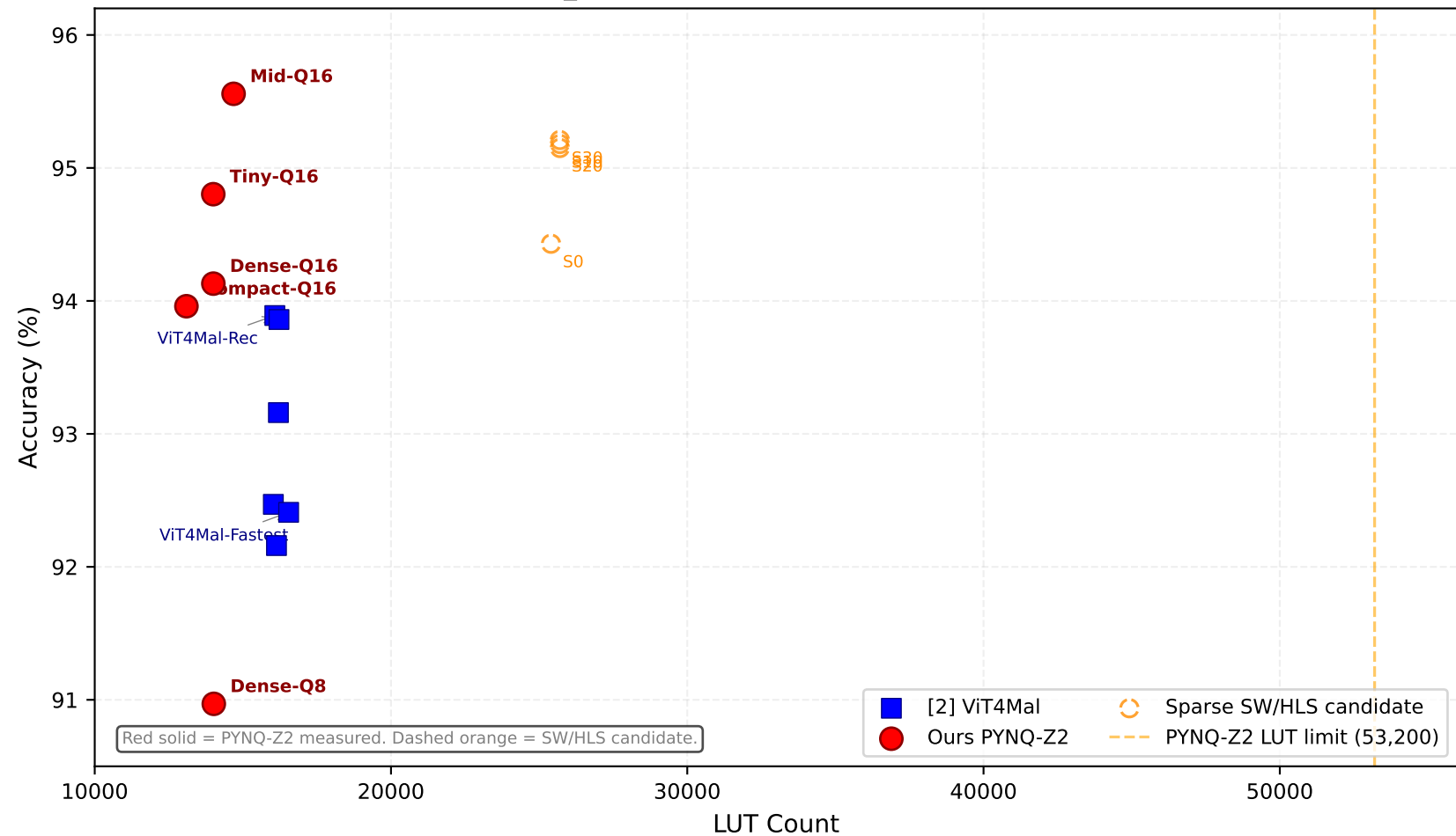
IMG_DS Pareto Frontier: Accuracy vs LUT
