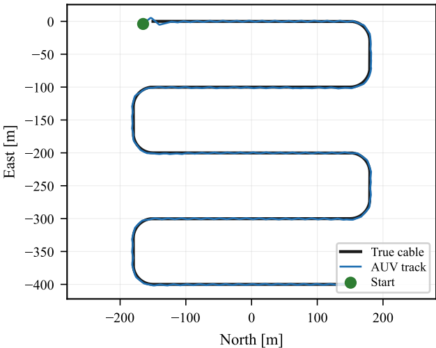
Trajectory vs. true cable
