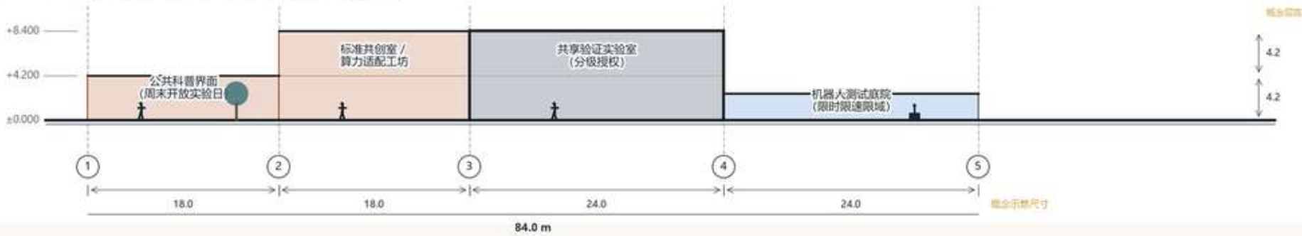
A—A' | 主剖面：科普界面—共创—实验室—测试庭院
