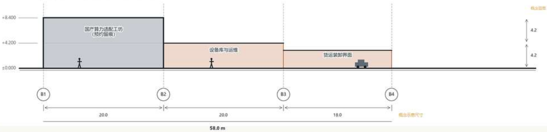
B—B' | 补充剖面：算力工坊—设备后勤—货运界面
