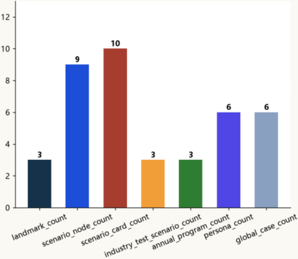
计数类指标 (编号对象见正文)
