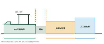
1:200 典型剖面 | 公共路径与试验湾物理分离
