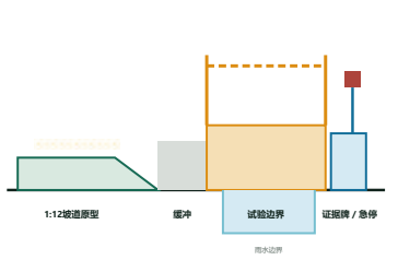
1:50 节点 | 坡道、盲道、可拆边界与雨水
