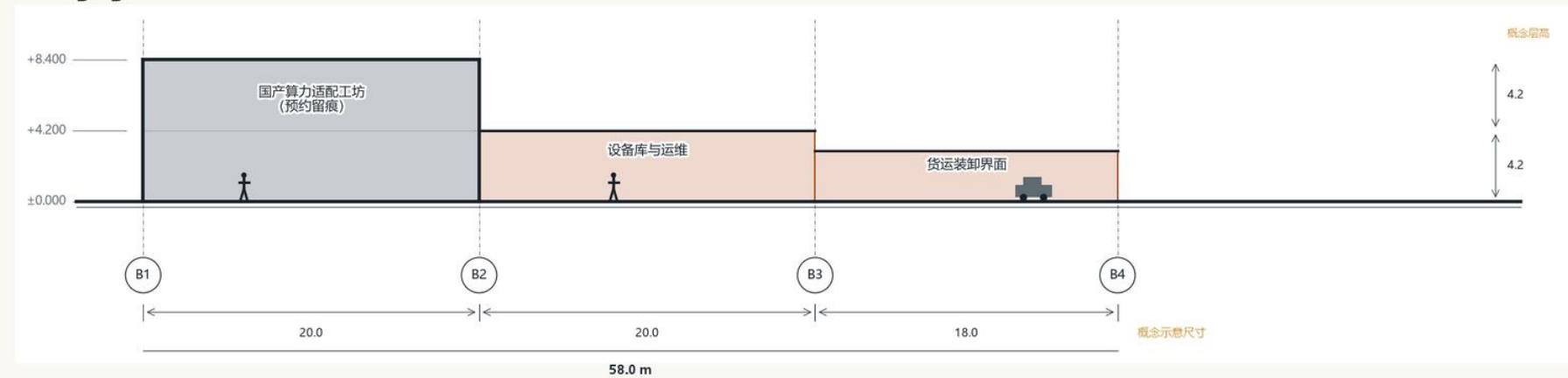
补充剖面：算力工坊—设备后勤—货运界面
