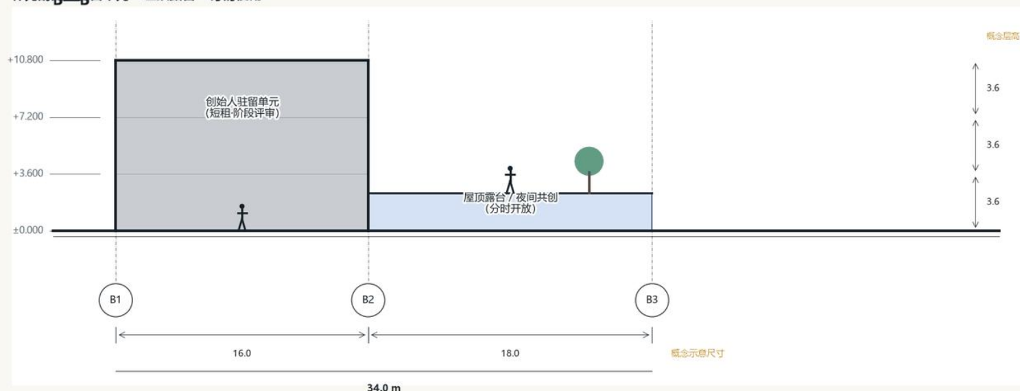
补充剖面：驻留单元—屋顶露台—分时使用
