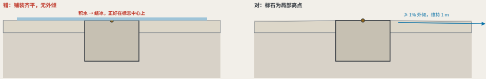
铺装齐平且不找坡：九月合拢，一月是人行道上唯一一块冰 坡度按真实比例绘制：1% 在 1 m 上是 10 mm，在这个比例下几乎看不见——看不见的坡度，现场也没有人会去查，而图上每一个尺寸都还是满足的。
