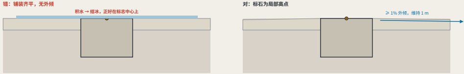
铺装齐平且不找坡：九月合拢，一月是人行道上唯一一块冰 坡度按真实比例绘制：1% 在 1 m 上是 10 mm，在这个比例下几乎看不见——看不见的坡度，现场也没有人会去查，而图上每一个尺寸都还是满足的。
