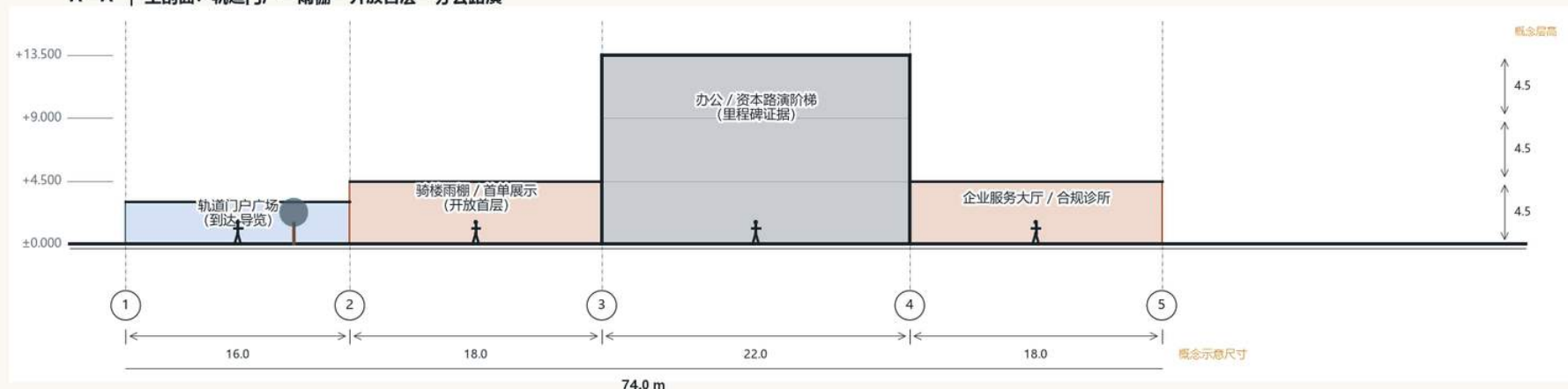
A—A' | 主剖面：轨道门户—雨棚—开放首层—办公路演
