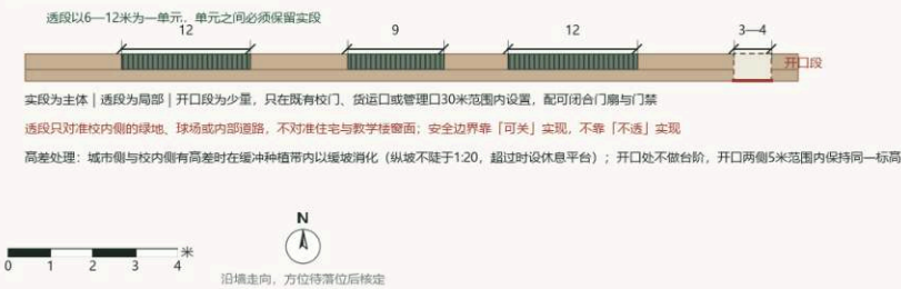
断面 ORI-1 · 校园围墙界面「透而不破」（概念断面示意）
