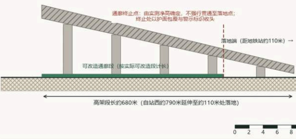
概念断面示意，不含工程结论；宽度为分配意向而非道路红线；待专业团队按现行标准核定。
