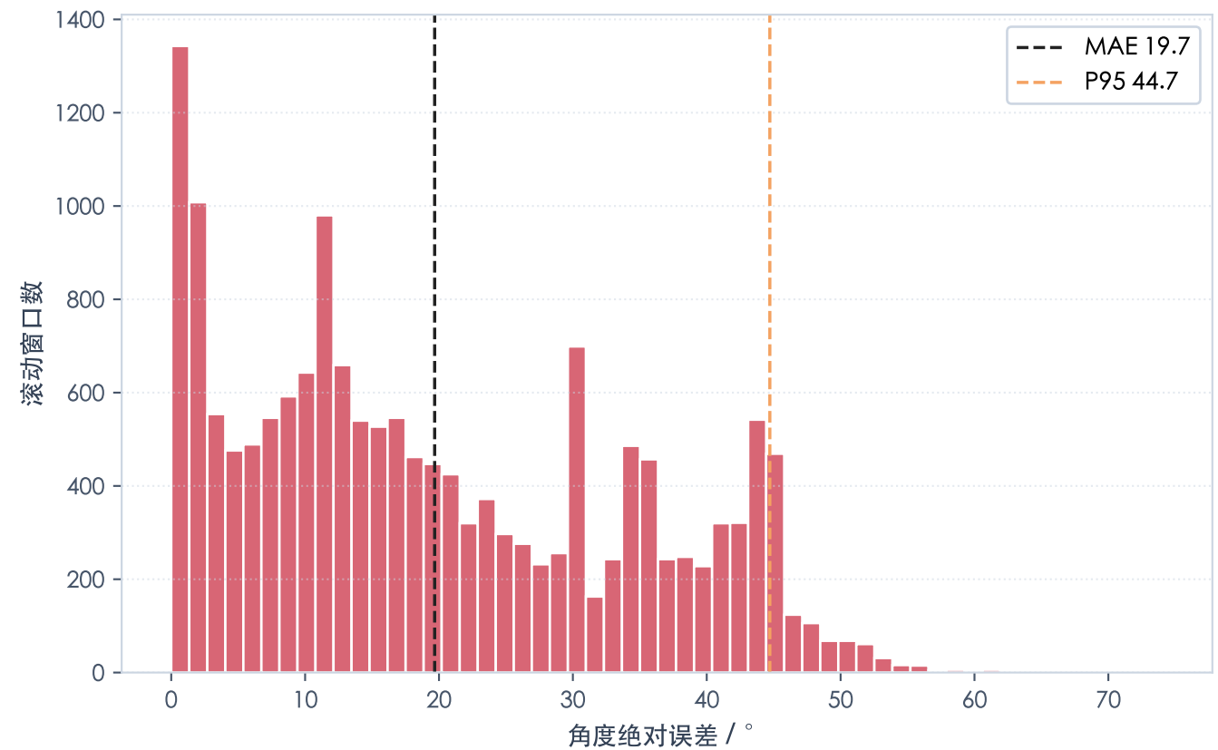
实际 0.8 s 滚动窗口误差分布 / CDF (n=16,931) 四站 190 mm · 2026-08-01 实测 · 整物理点留出验证
