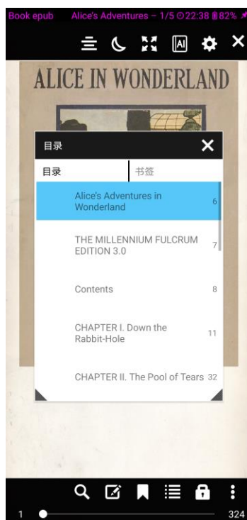
图 7 目录面板
