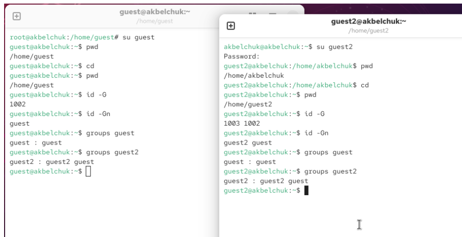
Рис. 2.2: Информация о пользователях
