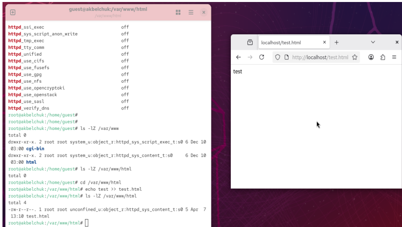
Рисунок 2: создание html-файла и доступ по http
