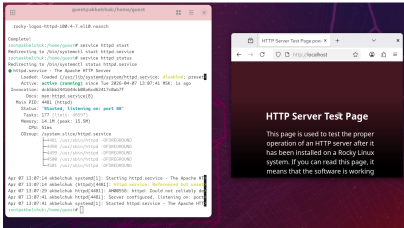
Рисунок 1: запуск http
