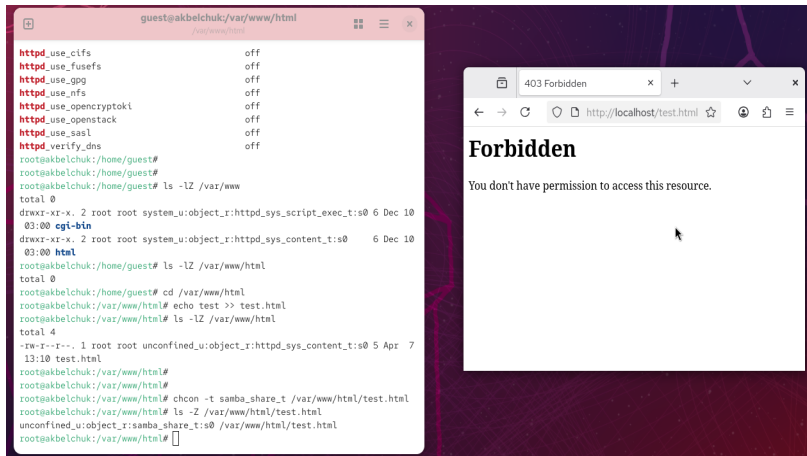
Рисунок 3: ошибка доступа после изменения контекста
