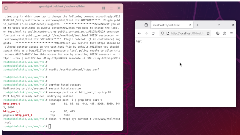
Рисунок 4: доступ по http на 81 порт
