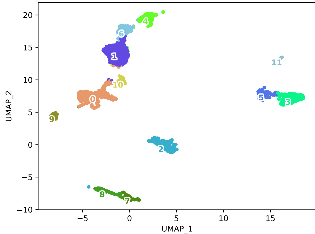
leiden_10_0.6
