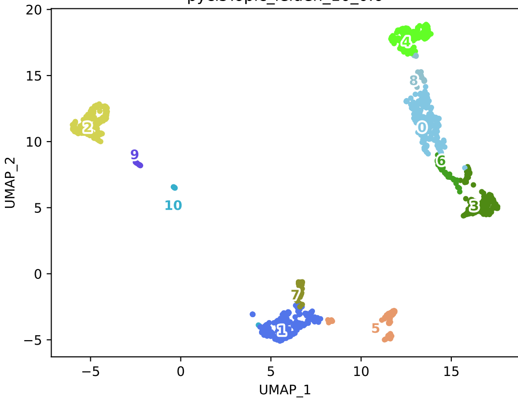
pycisTopic_leiden_10_0.6
