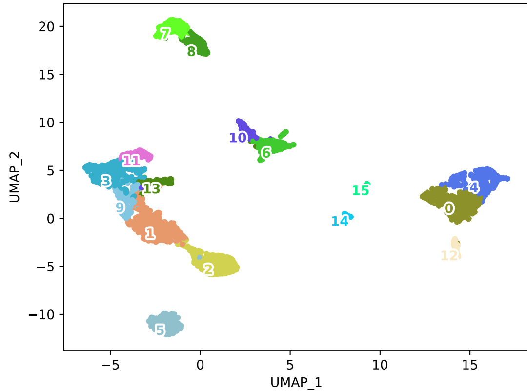
pycistopic_leiden_10_0.6
