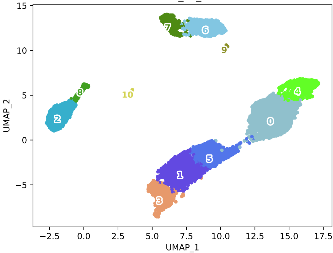
leiden_10_0.6
