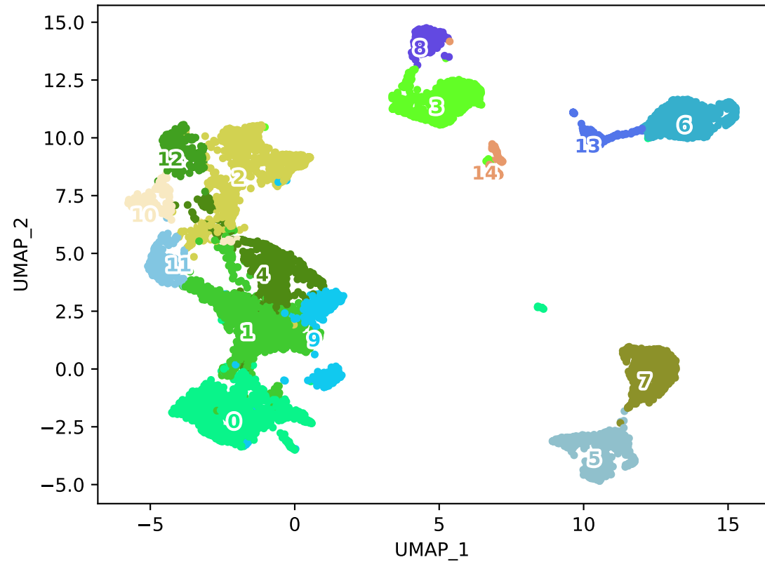
pycisTopic_leiden_10_0.6
