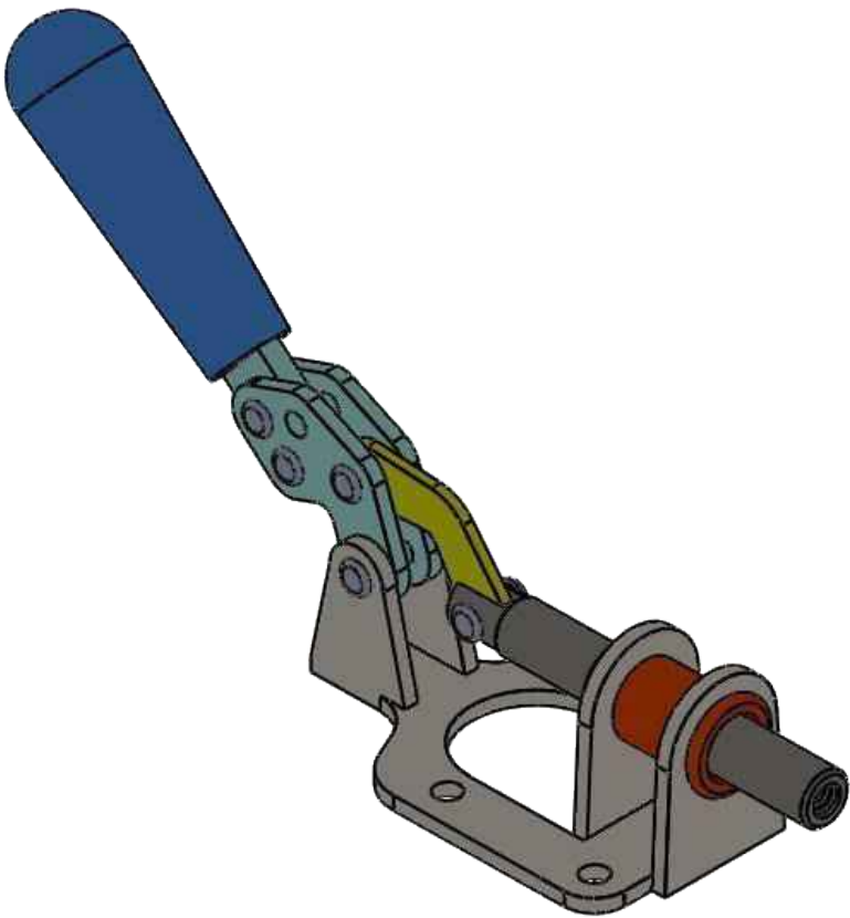
(1 : 1.4) ISOMETRIC
