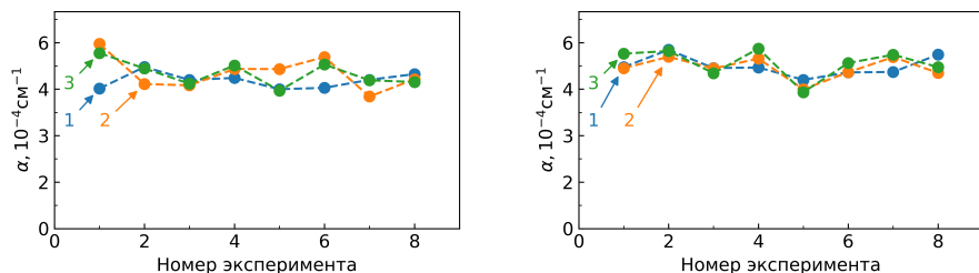
Рисунок 14 — Коэффициент оптического поглощения, определённый тремя методиками: 1 — экспоненциальный, 2 — импульсный, 3 — градиентный. Слева: без поправок, справа: совместный учёт поправок.
