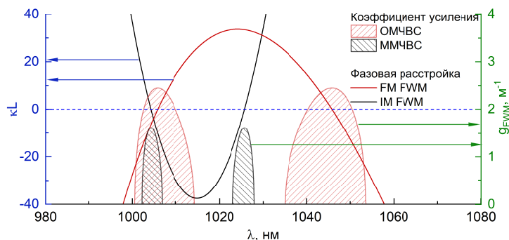
Рисунок 6 — Рассчитанная волновая расстройка (сплошные линии, левая шкала) и спектры усиления (затенённые области, правая шкала) для ОМЧВС (красный) и ММЧВС (чёрный). Длина ОВ доставки: L = 4 м.
