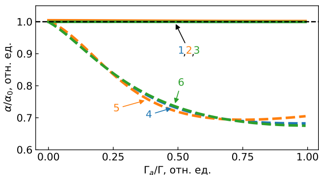
Рисунок 12 — Зависимость погрешности определения коэффициента поглощения от отношения скоростей теплоотдачи окружающей среды \Gamma_a и кристалла \Gamma . Кривые 1–3 — методы с учётом поправки; кривые 4–6 — без коррекции.
