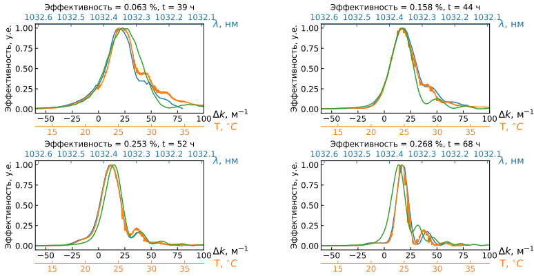
Рисунок 10 — КФС, измеренные на различных этапах записи \chi^{(2)} -решётки. Синие и оранжевые кривые — спектральный и температурный фазовые синхронизмы соответственно, зелёные — моделирование.
