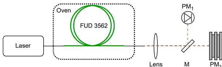
Рисунок 8 — Схема экспериментальной установки
