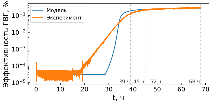
Рисунок 9 — Кинетика эффективности ГВГ в процессе формирования \chi^{(2)} -решётки (оранжевая кривая: эксперимент, синяя кривая: моделирование). Отмечены моменты времени, в которые проводились измерения КФС.
