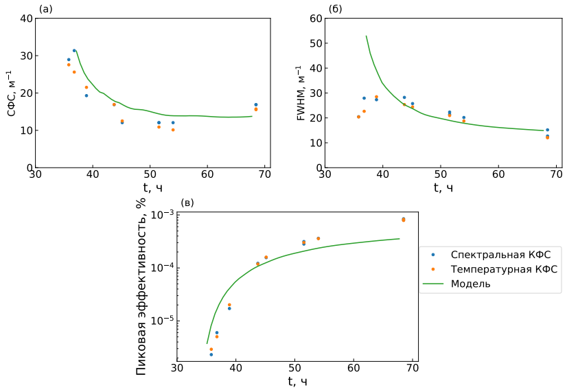
Рисунок 11 — Временные зависимости сдвига фазового синхронизма (СФС) (а), ширины кривой на половине высоты (FWHM) (б) и пиковой эффективности (в). Синие и оранжевые точки — эксперимент, зелёные кривые — моделирование.
