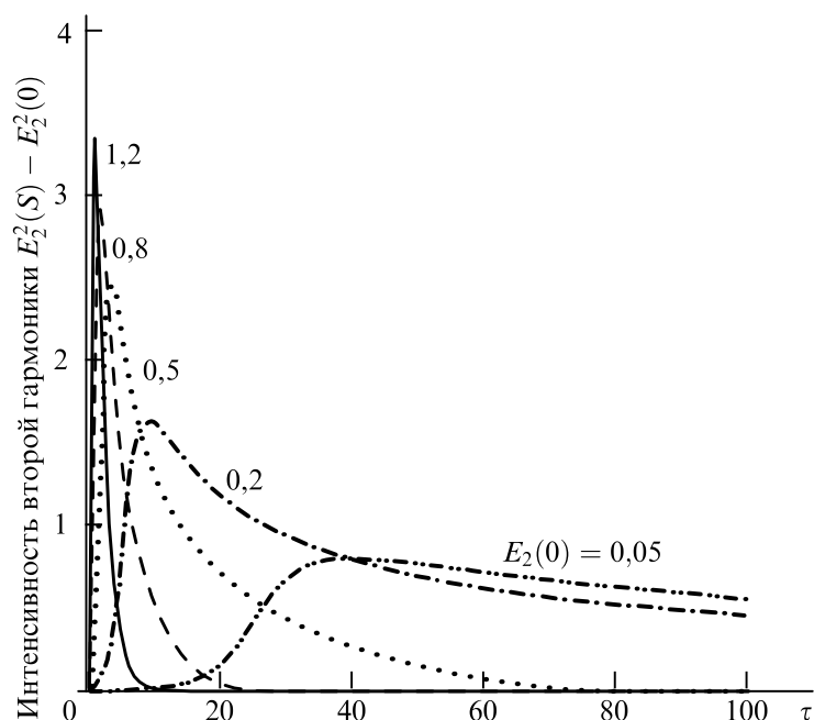
Рисунок 1.8 — Временная зависимость выходного сигнала второй гармоники для разных амплитуд входного сигнала. Из работы [67].
