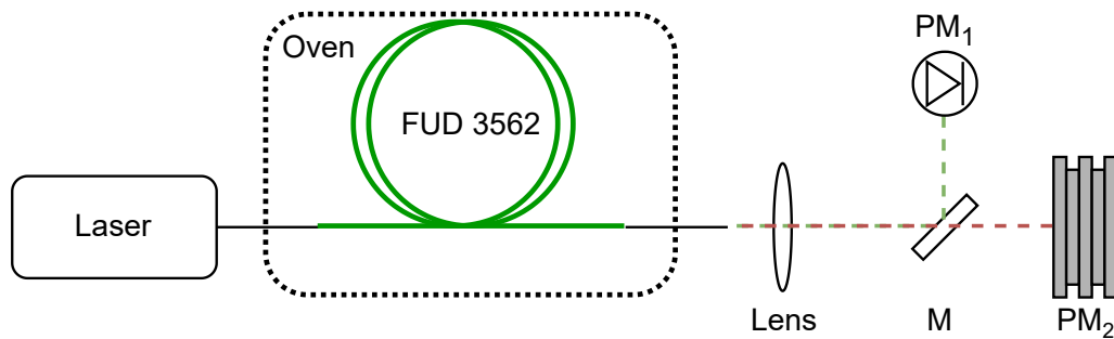
Рисунок 3.1 — Схема экспериментальной установки по исследованию КФС в условиях записи решётки нелинейной квадратичной восприимчивости. Чёрные участки ОВ: негерманосиликатное ОВ, в котором генерация второй гармоники пренебрежимо мала. М: набор дихроичных зеркал для разделения волн накачки и второй гармоники; PM_1 , PM_2 : фотодиодный и тепловой измерители мощности соответственно.
