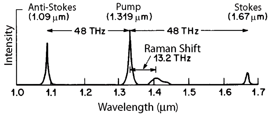
Рисунок 1.3 — Спектр на выходе одномодового ОВ при накачке излучением с длиной волны 1.319 мкм. Наблюдаются стокова компонента на 1.67 мкм и анти-стоксова на 1.09 мкм (из работы [52]).
