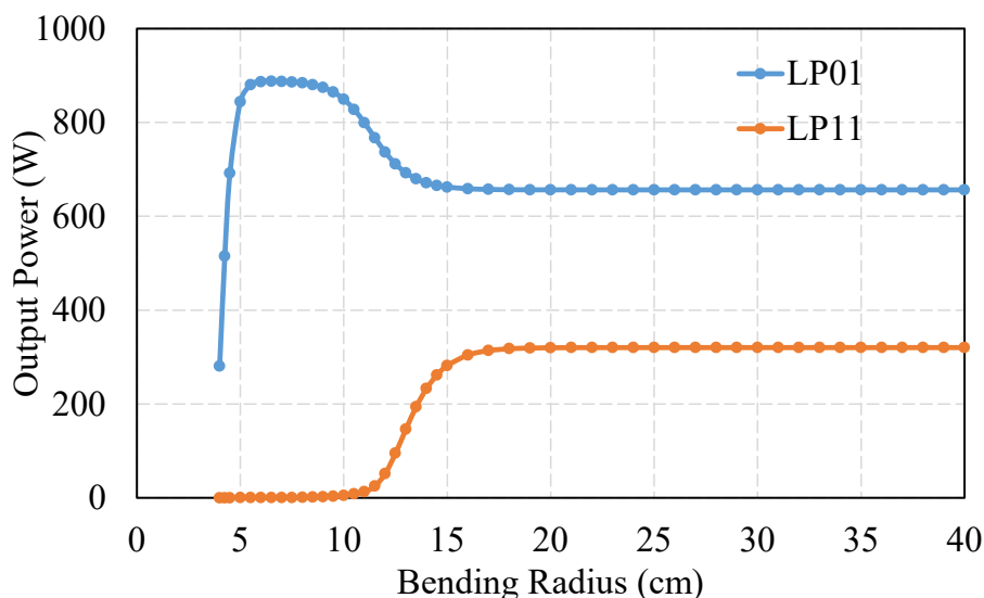
Рисунок 1.5 — Расчётная зависимость выходной мощности мод LP_{01} и LP_{11} от радиуса изгиба. Из работы [55].
